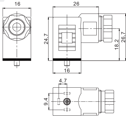
Konektor řady: 43650C DIN C
