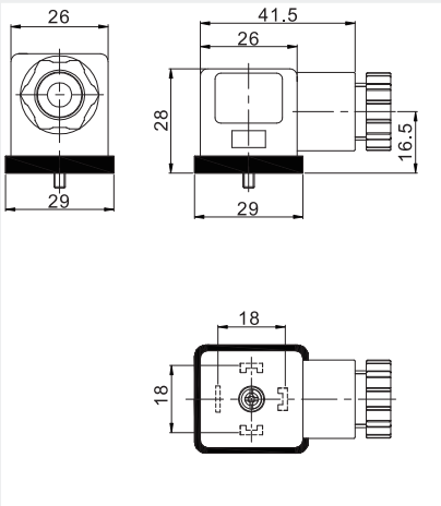
Konektor řady: 43650A Tvar A
